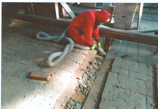
Trámový strop
